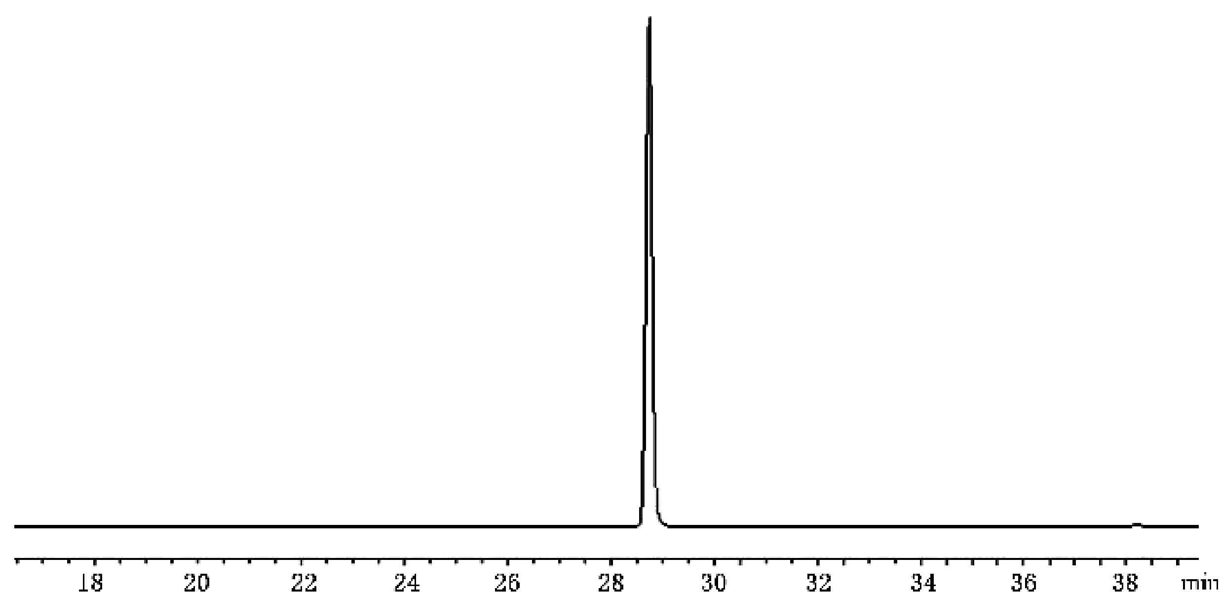
图 E.1 苯并[a]芘参考色谱图
