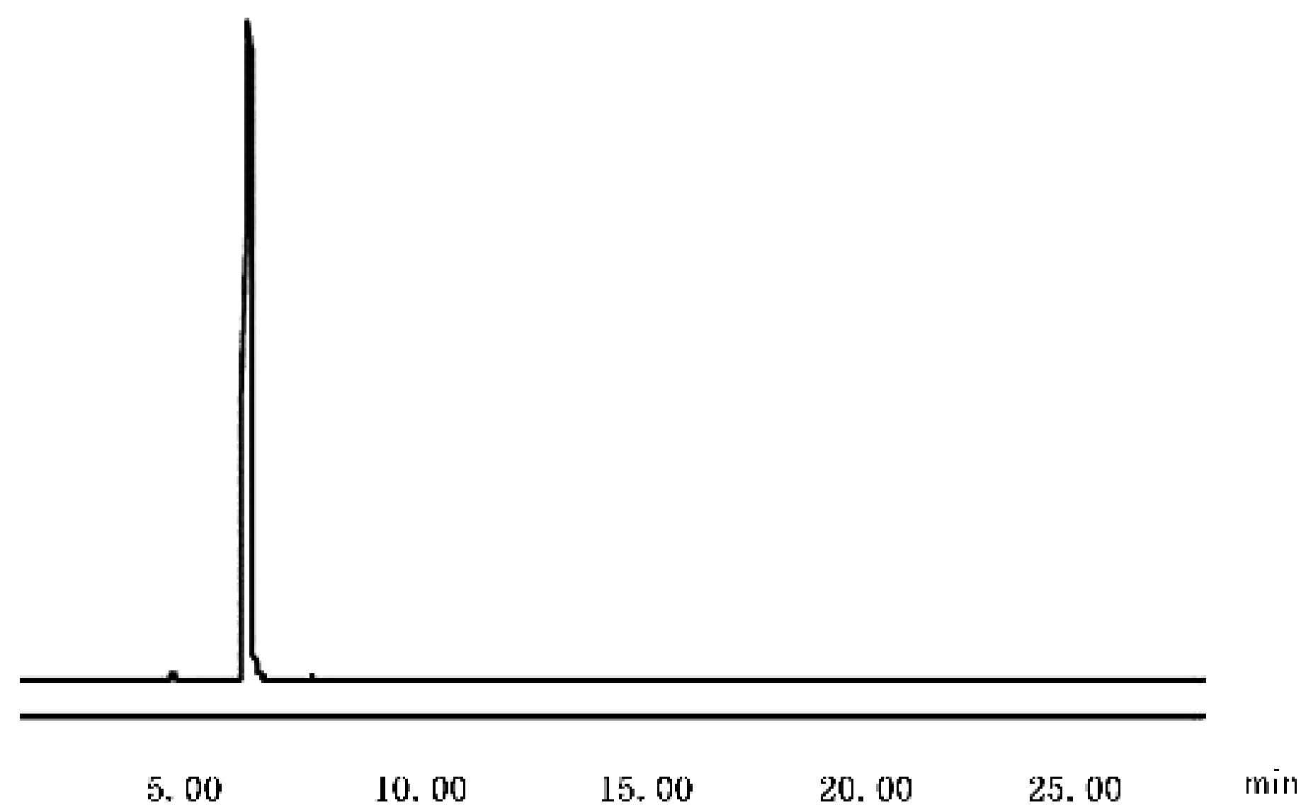
图 B.1 甲醛-2,4-二硝基苯腈参考色谱图
